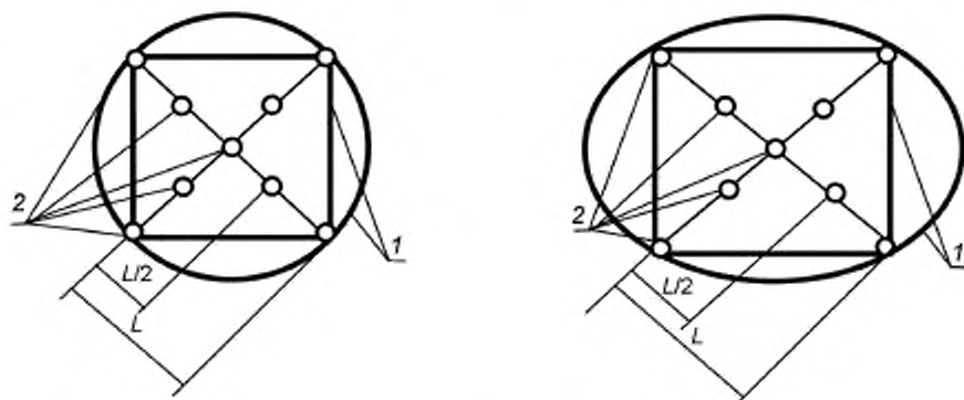
Рисунок 1 — Схема расположения модельных очагов пожара
